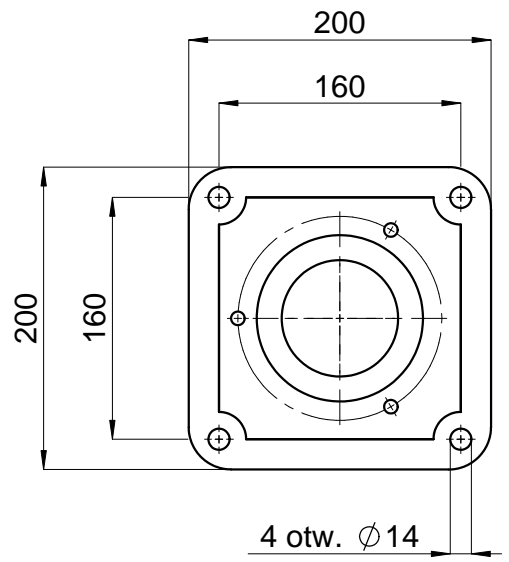
Widok „W”
